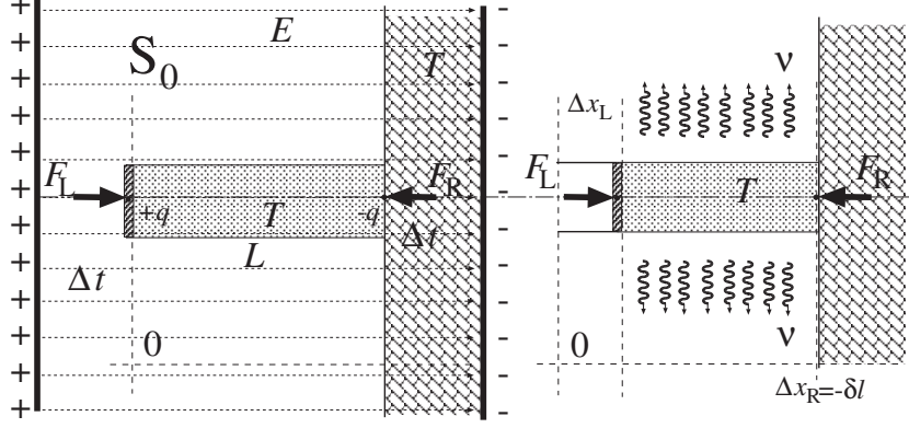
Figura 4: Gas a temperatura T encerrado en un cilindro de paredes diatermas, y dotado de un émbolo, que es comprimido bajo la acción de una fuerza F_L = qE que actúa sobre el émbolo debido a la interacción de una carga q depositada sobre el émbolo con un campo eléctrico E entre las placas de un condensador cargado, que se desplaza \Delta x_L . La base del cilindro, cerrado, se apoya en una pared. Sobre esta base, en la que hay depositada una carga -q , se aplica una fuerza F_R = -qE , con desplazamiento asociado \Delta x_R = -\delta l . Durante el proceso de compresión, se emiten fotones a un foco térmico a temperatura T . El proceso de compresión isoterma se observa desde el referencial S_0 en que el sistema se encuentra en reposo. Las fuerzas se aplican simultáneamente y el conjunto de fotones emitidos tienen momento lineal total nulo.
