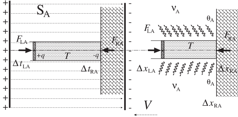
Figura 6: Proceso de compresión isoterma dado en Fig. 4, descrito desde el punto de vista de un observador en el referencial S_A en configuración estándar, con velocidad V respecto del referencial S_0 . La fuerza F_{RA} tiene asociado el desplazamiento \Delta x_{RA} y la fuerza F_{LA} tiene asociado el desplazamiento \Delta x_{LA} . Las fuerzas F_{RA} y F_{LA} no se aplican ni simultáneamente ni durante el mismo intervalo de tiempo y se tiene un impulso neto aplicado sobre el gas. Los fotones se emiten con frecuencia \nu_A y formando un ángulo \theta_A con la horizontal. El calor Q_A lleva asociado momento lineal no nulo.
