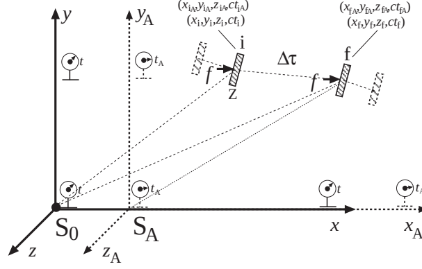
Figura 7: Referenciales S_0 y S_A en configuración estándar. (i) Una fuerza f comienza a actuar sobre un cuerpo Z . Suceso inicial, subíndice i en ambos referenciales, (f) suceso final, la fuerza f deja de actuar sobre Z . El tiempo \Delta\tau es el intervalo de tiempo propio de Z ([63], Sec. 2.9) entre los sucesos inicial y final. Los 4-vectores suceso inicial, x_i^\mu = \{x_i, y_i, z_i, ct_i\} en S y x_{iA}^\mu = \{x_{iA}, y_{iA}, z_{iA}, ct_{iA}\} en S_A y suceso final, x_f^\mu = \{x_f, y_f, z_f, ct_f\} en S y x_{fA}^\mu = \{x_{fA}, y_{fA}, z_{fA}, ct_{fA}\} en S_A se relacionan entre sí como x_{iA}^\mu = \mathcal{L}_\nu^\mu(V)x_i^\nu y x_{fA}^\mu = \mathcal{L}_\nu^\mu(V)x_f^\nu , respectivamente, donde \mathcal{L}_\nu^\mu(V) es la matriz de la transformación de Lorentz para la configuración estándar.
