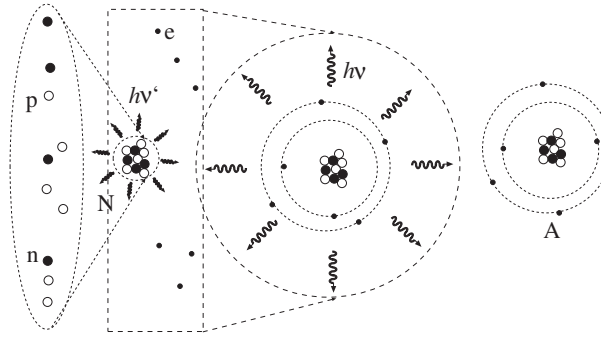
Figura 1: Formación de un átomo (A) a partir de su núcleo (N), previamente formado a partir de protones y neutrones, y de electrones (e), situados previamente en el infinito. La inercia del núcleo \mathcal{M}_N = U_N c^{-2} es menor que la suma de las inercias de sus componentes \mathcal{U}_N = 6m_p c^2 + 4m_n , \mathcal{M}_A = \mathcal{U}_N c^{-2} - |\Delta \mathcal{M}_N| , debido a la energía liberada en forma de fotones \Delta \mathcal{M}_N = -(8h\nu') c^{-2} cuando se forma el núcleo. La inercia del átomo \mathcal{M}_A = U_A c^{-2} es menor que la suma de las inercias de sus componentes \mathcal{U} = 6m_e c^2 + \mathcal{M}_N c^2 , \mathcal{M}_A = \mathcal{U}_A c^{-2} - |\Delta \mathcal{M}_A| , debido a la energía liberada en forma de fotones \Delta \mathcal{M}_A = -(8h\nu) c^{-2} cuando se forma el átomo.
