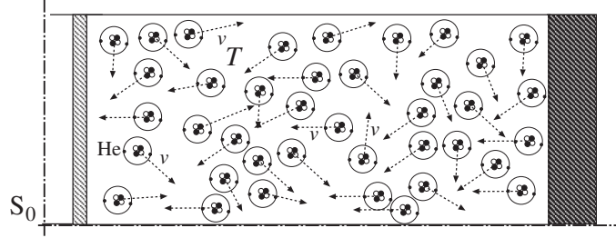
Figura 5: Sistema formado por (1 mol de) átomos de He, a temperatura T . En la aproximación mono-cinética, cada átomo se mueve con velocidad |\mathbf{v}| = v . En el referencial S_0 el momento lineal total del sistema es cero. Cada átomo tiene una cierta energía cinética K = [\gamma(v) - 1]u , donde v(T) = aT^{1/2} .
