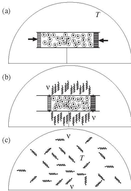
FIGURA 3. (a) Un gas contenido en un cilindro es comprimido bajo la acción de dos émbolos dentro de una cavidad a temperatura T (proceso isoterma), respecto de la cual se mantiene en reposo (su centro de masas se encuentra en reposo en los estados inicial y final de equilibrio termodinámico). (b) Durante el proceso de compresión se emiten fotones de frecuencia \nu = \nu(T) con momento lineal total nulo. (c) El calor emitido durante la compresión se modeliza como energía asociada a la radiación formada por todos los fotones emitidos contenida en la cavidad U_F(T) = Nh\nu (cambiada de signo).
