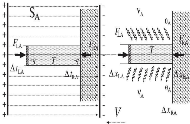
FIGURA 6. Proceso de compresión isoterma dado en Fig. 4, descrito desde el punto de vista de un observador en el referencial S_A en configuración estándar, con velocidad V respecto del referencial S_0 . La fuerza F_{RA} tiene asociado el desplazamiento \Delta x_{RA} y la fuerza F_{LA} tiene asociado el desplazamiento \Delta x_{LA} . Las fuerzas F_{RA} y F_{LA} no se aplican ni simultáneamente ni durante el mismo intervalo de tiempo y se tiene un impulso neto aplicado sobre el gas. Los fotones se emiten con frecuencia \nu_A y formando un ángulo \theta_A con la horizontal. El calor Q_A lleva asociado momento lineal no nulo.
