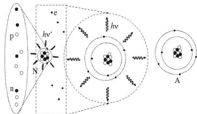
FIGURA 1. Formación de un átomo (A) a partir de su núcleo (N), previamente formado a partir de protones, neutrones, y de electrones (e), situados previamente en el infinito. La inercia del núcleo M_N = U_{NC} c^{-2} es menor que la suma de las inercias de sus componentes U_N = 6m_p c^2 + 4m_n , M_A = U_{NC} c^{-2} - |\Delta M_N| , debido a la energía liberada en forma de fotones \Delta M_N = -(8h\nu') c^{-2} cuando se forma el núcleo. La inercia del átomo M_A = U_{AC} c^{-2} es menor que la suma de las inercias de sus componentes U = 6m_e c^2 + M_N c^2 , M_A = U_{AC} c^{-2} - |\Delta M_A| , debido a la energía liberada en forma de fotones \Delta M_A = -(8h\nu) c^{-2} cuando se forma el átomo.
