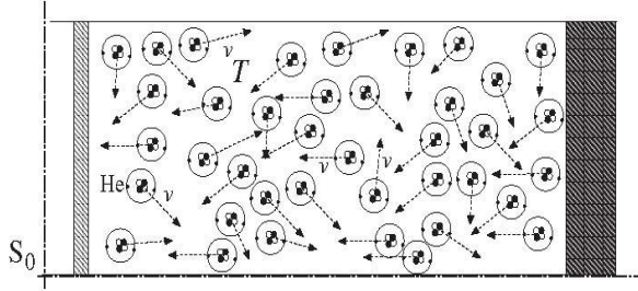
FIGURA 5. Sistema formado por (1 mol de) átomos de He, a temperatura T . En la aproximación mono-cinética, cada átomo se mueve con velocidad |\mathbf{v}| = v . En el referencial S_0 el momento lineal total del sistema es cero. Cada átomo tiene una cierta energía cinética K = \gamma(v) - 1 u , donde v(T) = aT^{1/2} .
