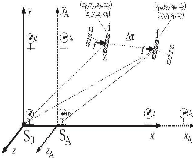
FIGURA 7. Referenciales S_0 y S_A en configuración estándar. (i) Una fuerza f comienza a actuar sobre un cuerpo Z . Suceso inicial, subíndice i en ambos referenciales, (f) suceso final, la fuerza f deja de actuar sobre Z . El tiempo \Delta\tau es el intervalo de tiempo propio de Z ([63], Sec. 2.9) entre los sucesos inicial y final. Los 4-vectores suceso inicial, x_i^\mu = \{x_i, y_i, z_i, ct_i\} en S y x_{iA}^\mu = \{x_{iA}, y_{iA}, z_{iA}, ct_{iA}\} en S_A y suceso final, x_f^\mu = \{x_f, y_f, z_f, ct_f\} en S y x_{fA}^\mu = \{x_{fA}, y_{fA}, z_{fA}, ct_{fA}\} en S_A se relacionan entre sí como x_{iA}^\mu = L_\nu^\mu(V) x_i^\nu y x_{fA}^\mu = L_\nu^\mu(V) x_f^\nu , respectivamente, donde L_\nu^\mu(V) es la matriz de la formación de Lorentz para la configuración estándar.
