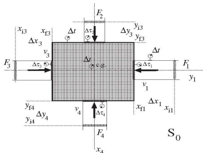
FIGURA 2. Fuerzas F_k ( k = 1, 2, 3, 4 ) aplicadas, con impulso y torque nulos, sobre un sistema deformable durante un intervalo de tiempo \Delta t medido en el referencial S_0 en el que el sistema (c.g.) se encuentra en reposo, al menos, en sus estados de equilibrio inicial y final. Cada émbolo, con desplazamiento \Delta r_k = r_{fk} - r_{ik} ( r \equiv x, y, z ) y desplazado con velocidad v_k , tiene su particular tiempo propio \Delta \tau_k . El 4-vector velocidad v_k^\mu asociado al desplazamiento del k -ésimo émbolo viene dado por v_k^\mu = \Delta r_k^\mu / \Delta \tau , con \Delta r_k^\mu = r_{fk}^\mu - r_{ik}^\mu = \Delta x_k, \Delta y_k, \Delta z_k, c \Delta t .
