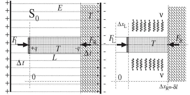
FIGURA 4. Gas a temperatura T encerrado en un cilindro de paredes diatermas, y dotado de un émbolo, que es comprimido bajo la acción de una fuerza F_L = qE que actúa sobre el émbolo debido a la interacción de una carga q depositada sobre el émbolo con un campo eléctrico E entre las placas de un condensador cargado, que se desplaza \Delta x_L . La base del cilindro, cerrado, se apoya en una pared. Sobre esta base, en la que hay depositada una carga -q , se aplica una fuerza F_R = -qE , con desplazamiento asociado \Delta x_R = -\delta l . Durante el proceso de compresión, se emiten fotones a un foco térmico a temperatura T . El proceso de compresión isoterma se observa desde el referencial S_0 en que el sistema se encuentra en reposo. Las fuerzas se aplican simultáneamente y el conjunto de fotones emitidos tienen momento lineal total nulo.
