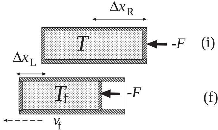
Figura 2: (i) Sobre un gas de Van der Waals encerrado en un cilindro dotado de un émbolo, a temperatura T , se aplica una fuerza -F sobre el émbolo, sin ninguna otra fuerza aplicada. (f) Durante el intervalo de tiempo \Delta t , el émbolo se mueve una distancia \Delta x_R , mientras que el extremo cerrado del cilindro se desplaza una distancia \Delta x_L . El sistema conjunto adquiere una velocidad v_f . El proceso se puede considerar adiabático (A) o isotermo (I).
