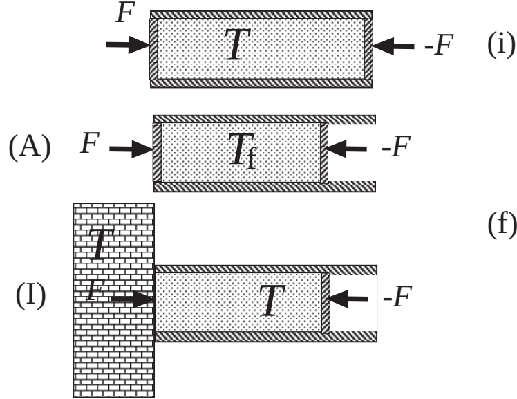
Figura 1: (i) Sobre un gas de Van der Waals encerrado en un cilindro dotado de un émbolo, a temperatura T , se aplica una fuerza -F sobre el émbolo. (f) El proceso de compresión se describe como adiabático, (A), con el gas alcanzando una temperatura final T_f ; el proceso de compresión se describe como isoterma, (I), con el gas en contacto con un foco térmico a temperatura T .
