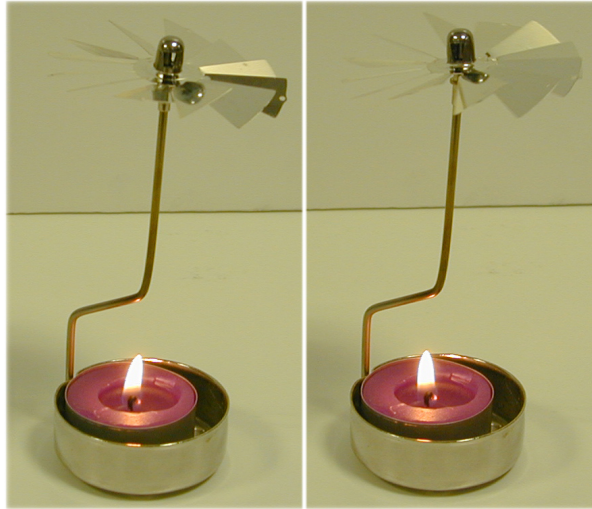
Figura 15: Molinete térmico . Apoyado sobre una punta, el aire caliente ascendente golpea sus álabes, cuya inclinación respecto de la vertical permite que, por reacción, se produzca el par de fuerzas que hace girar lo hace girar.
