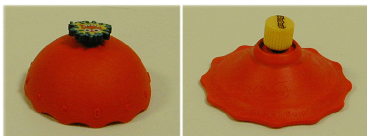
Figura 10: Resorte de caucho . Se trata de una cúpula hueca de caucho que permanece deformada si se la invierte. (i) En su posición normal. (d) Preparado para liberar la energía elástica y elevarse en vertical al ser dejado caer, haciéndole girar con la ayuda de la manilla, y chocar contra el suelo.
