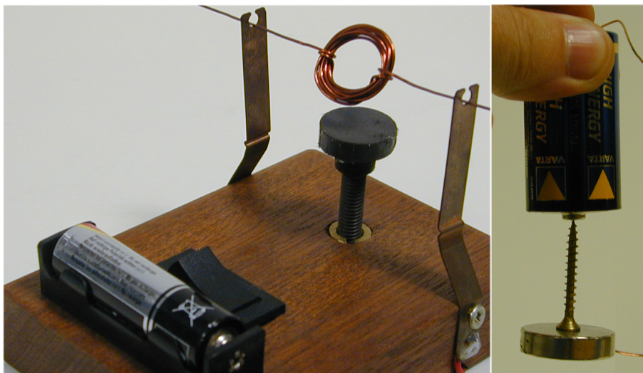
Figura 20: (i) Motor eléctrico simple . Cuando circula corriente por la pequeña bobina situada sobre el imán, ésta gira. (d) Motor Homopolar . Si se conecta el extremo superior de la pila con el borde del imán de neodimio con forma de disco, éste gira.
