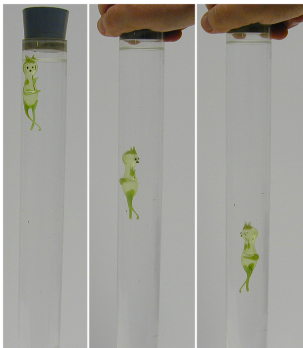
Figura 12: Ludió . La figurita con forma de diablillo, está dotada de un tubo capilar, en la cola del diablillo, y con una burbuja de aire atrapada en su interior, flota en el agua. Al apretar el tapón que cierra la probeta, el ludió termina por descender por debajo del nivel del líquido, alcanzando el fondo de ésta.
