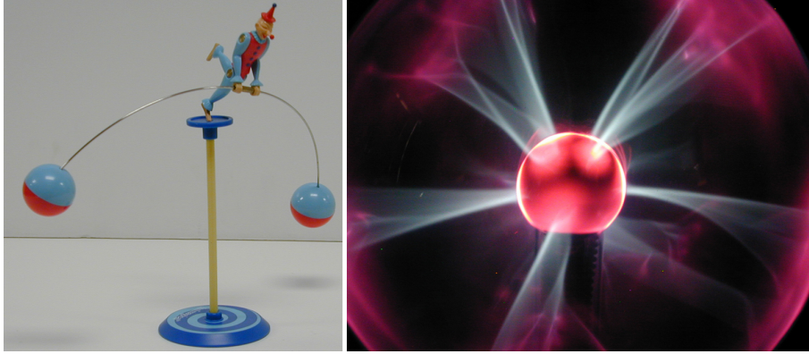
Figura 1: (i) Tentetieso . Sus contrapesos laterales consiguen que su centro de gravedad se sitúe por debajo de su punto de apoyo en la peana, proporcionándole la estabilidad que exhibe. (d) Lámpara de plasma . Conteniendo un gas a baja presión, en su centro se encuentra una bobina de Tesla capaz de generar altas tensiones, produciendo la ruptura dieléctrica del gas y la visualización del recorrido de los electrones.
