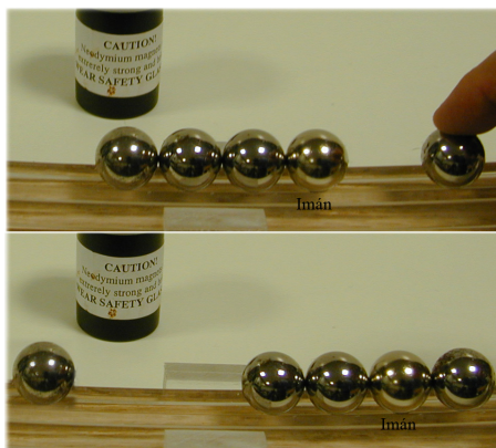
Figura 22: Cañón de Gauss . Cuatro bolas de acero, la cuarta es un imán de neodimio-boro-hierro, se colocan sobre un carril. Se deja libre una quinta bola, que es atraída por el imán. La primera bola sale despedida a gran velocidad, alcanza una altura importante y el restante conjunto de cuatro bolas, se desplaza moviéndose en sentido contrario (Tercera Ley de Newton).
