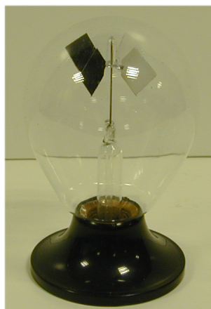
Figura 17: Radiómetro de Crookes . El radiómetro no funciona debido a la presión de radiación, la idea original de Crookes al construirlo, sino debido a un mecanismo de choques contra los bordes de los rombos, por lo que se necesita una pequeña cantidad de aire a baja presión. Si hubiera demasiado aire, el rozamiento haría que se detuviera el giro de las paletas.
