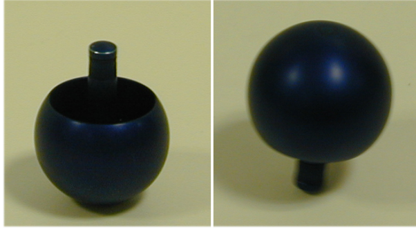
Figura 3: Tip-Top . Cuando esta peonza se ha invertido y gira sobre su vástago, la velocidad de rotación es menor que la velocidad de rotación cuando gira sobre la base esférica, pues al elevar su centro de gravedad parte de la energía cinética de rotación se ha invertido en energía potencial gravitatoria.
