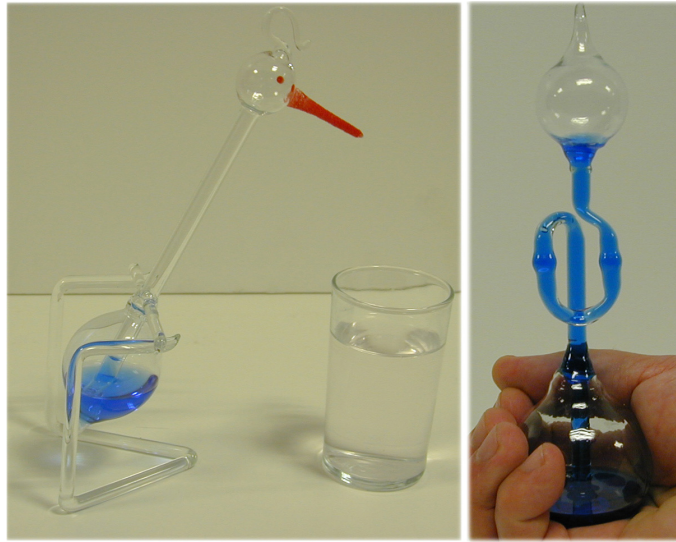
Figura 18: (i) Pájaro bebedor . El enfriamiento de su cabeza induce la diferencia de presiones suficiente como para que el líquido del cuerpo ascienda por el tubo central hasta su cabeza. (d) Hervidor de mano . Al calentar su base llena de líquido, la presión de vapor del líquido aumenta tanto que consigue elevarlo a través del tubo central hasta el bulbo superior.
