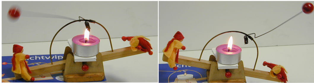
Figura 16: Balancín térmico . Con la espiral bimetálica situada sobre la llama, la esfera se desplaza hacia la derecha, haciendo girar el balancín y separando la espiral de la llama. Al enfriarse la espiral, la esfera de madera se desplaza hacia la izquierda, el balancín oscila hacia la izquierda y el muelle vuelve a situarse sobre la llama, cerrándose el ciclo.
