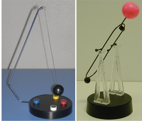
Figura 21: (i) Péndulo magnético . La bola del péndulo, que contiene una pieza de hierro, oscila caóticamente entre los imanes antes de detenerse. (d) Péndulo controlado electrónicamente . Al pasar cerca de la base, que oculta un electroimán controlado electrónicamente y una pila, recibe un impulso que compensa las pérdidas por rozamiento y le permite oscilar durante mucho tiempo.
