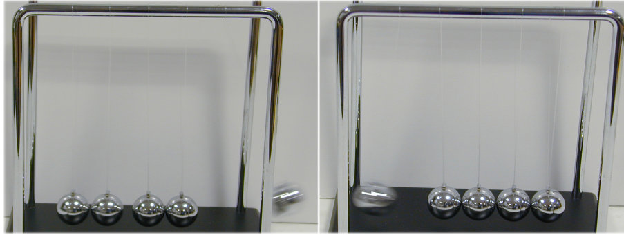
Figura 7: Cuna de Newton . Fue inventada por Willen J Gravesande (1688-1742) para estudiar la física de los choques. Las leyes de conservación del momento lineal y de conservación de la energía mecánica, implican que si una, dos, tres, etc., bolas son separadas hasta una cierta altura y luego dejadas caer, una, dos, tres, etc., bolas, respectivamente, serán desplazadas del otro lado de la cuna.
